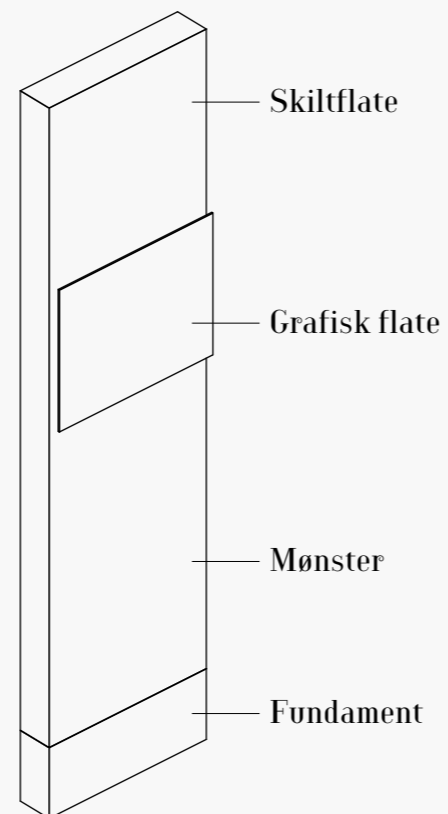
SR 3 a Skiltkiosk uten retningskilte
